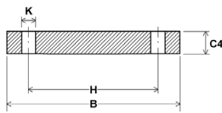
BLANK
