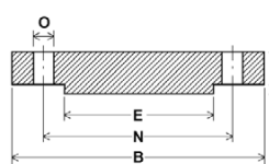
BLANK
